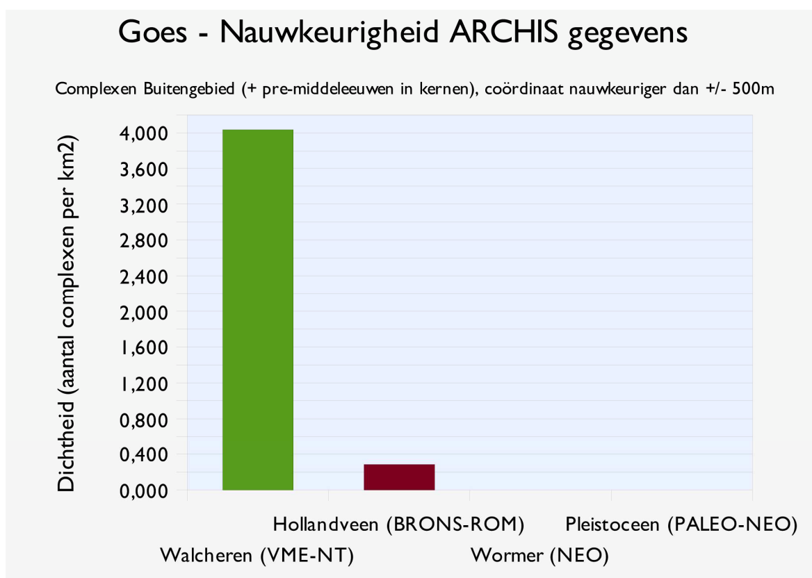
Afbeelding 2 Dichtheid van waarnemingen buiten de dorpskernen (nieuwe contour 1830). In de staafdiagrammen van de lagen voorafgaande aan de laag Walcheren (VME-NT) is niet het areaal in de berekening betrokken dat is geërodeerd door latere afzettingen.
